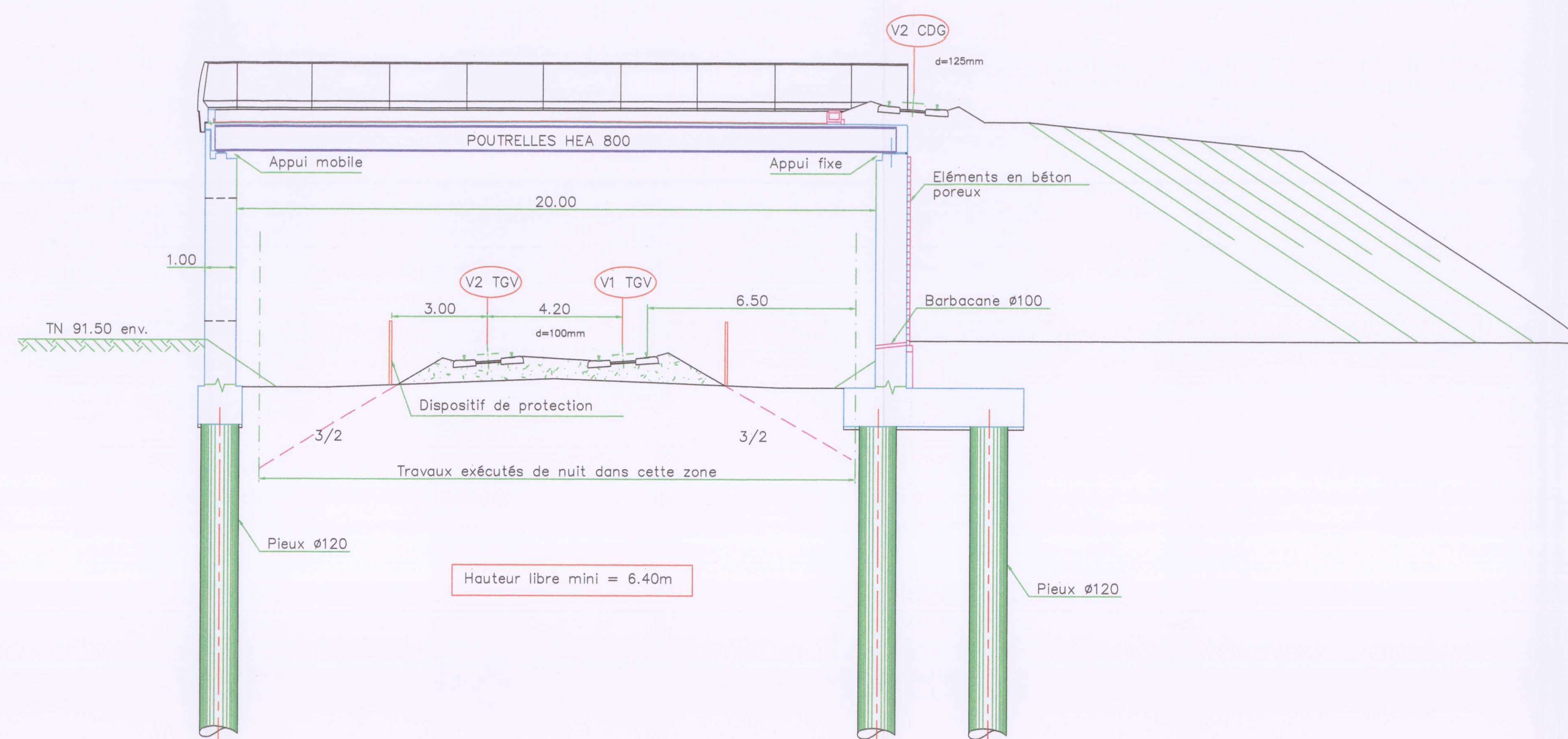
COUPE TRANSVERSALE B-B Ech : 1/100e
