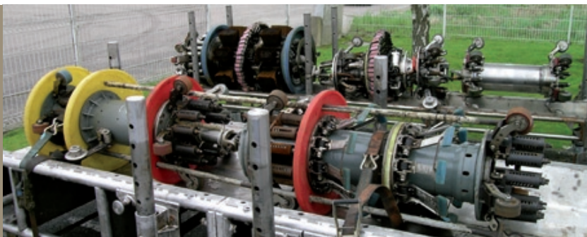
» Piston instrumenté
