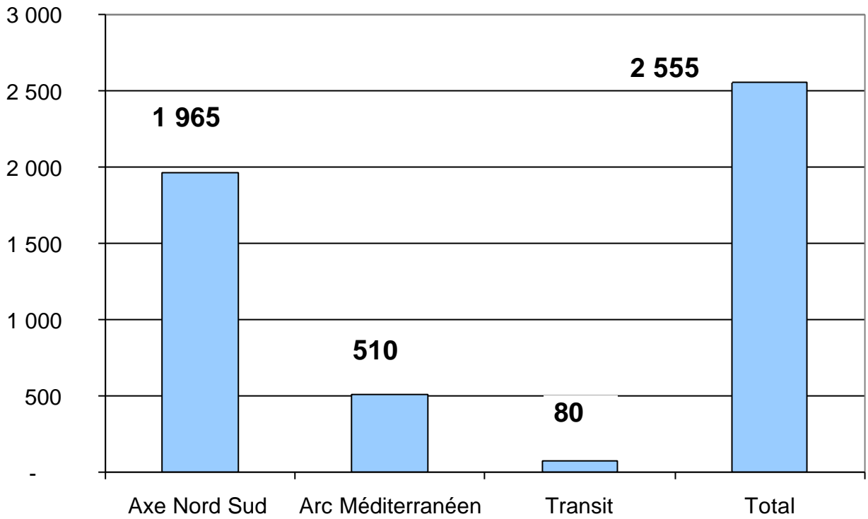
Figure 35 : Charges ferroviaires par sections
