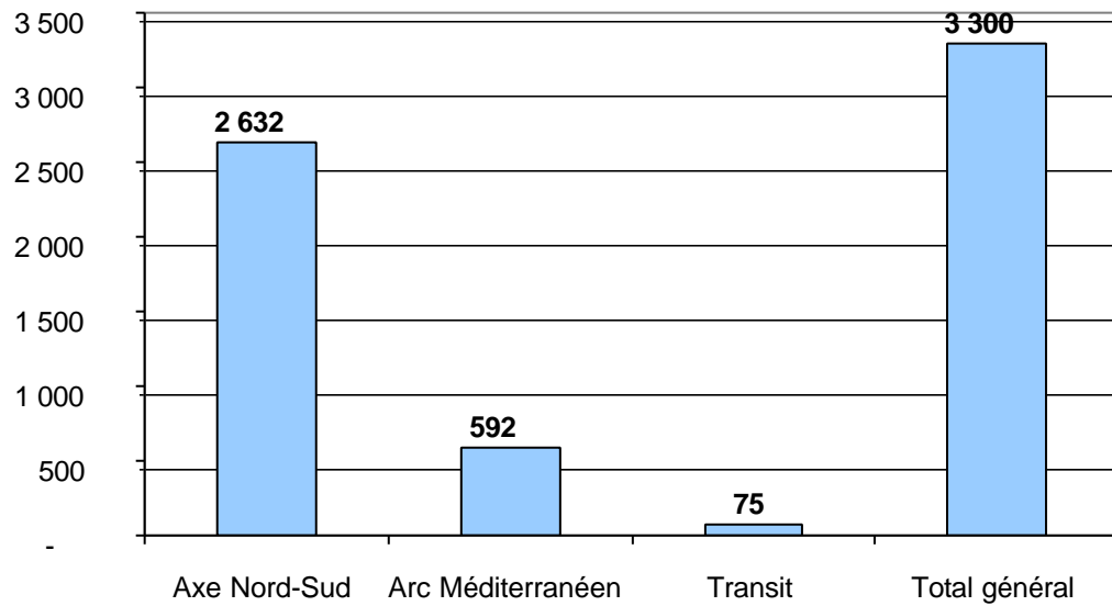
Figure 25 : Gain de trafic ferroviaire scénario de desserte à deux axes - Nord Arbois - A8 - Toulon Nord
