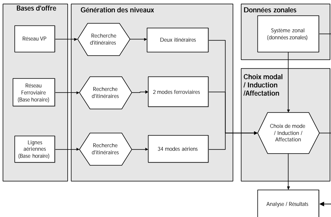
Figure 5 : Organigramme simplifié de la chaîne de traitement d'une situation d'étude
