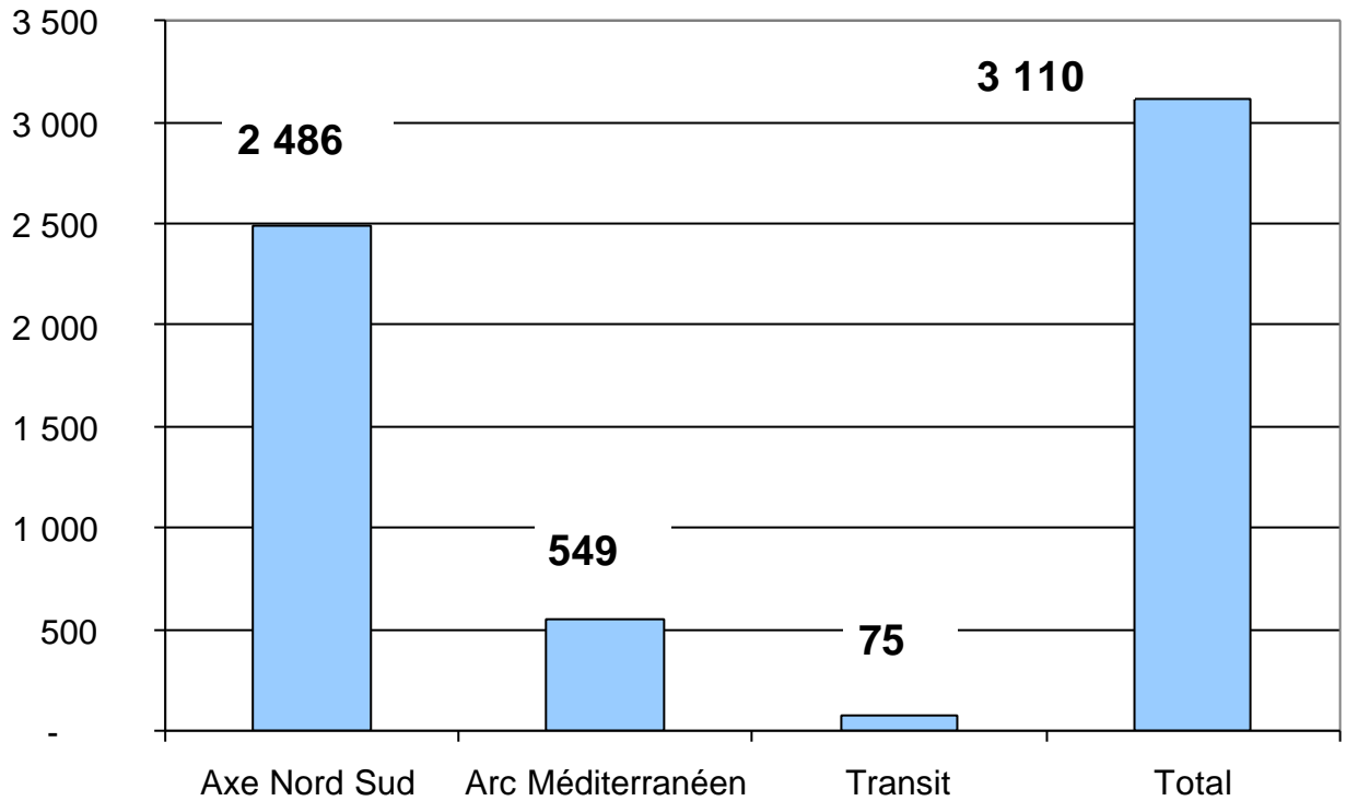
Figure 29 : Gain de trafic ferroviaire scénario de desserte à deux axes -Sud Arbois - Nord Toulon
