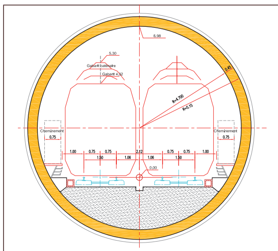
COUPE DE LA CONFIGURATION MONOTUBE DU TUNNEL
