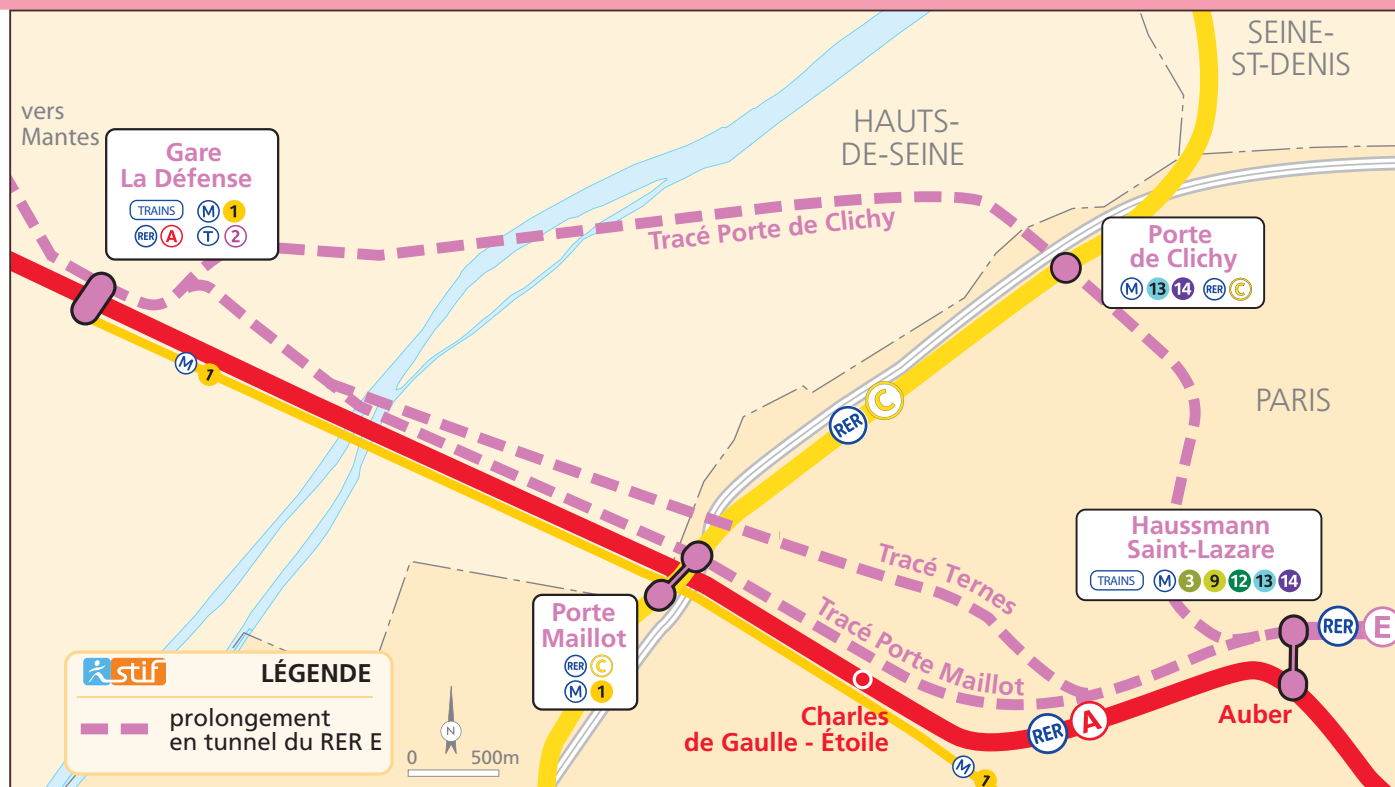
LES 3 VARIANTES DE TRACÉ ENTRE HAUSSMANN-SAINT- LAZARE ET LA DÉFENSE
