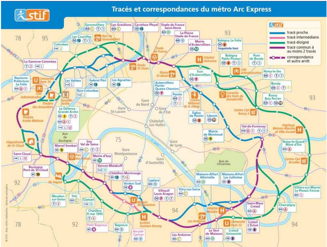
Carte 1 : Tracé modificatif du Projet Régional « Arc Express » du 15 novembre 2010
