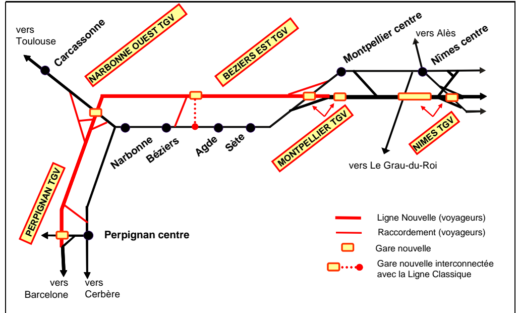
Figure 14 Schéma fonctionnel scénario A3 en phase 3
